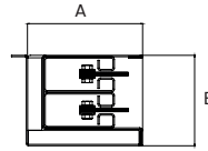
LATERAL GUÍA TORNILLOS A: 170 mm B: 130 mm
